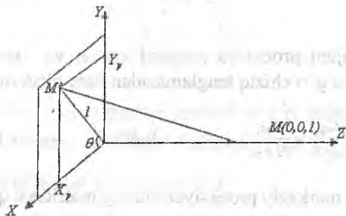
2.8-rasm. Qiya burchakli proeksiya.
