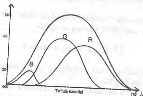
2.26-rasm. Ko'zning nisbiy ta'sirchanligi.
