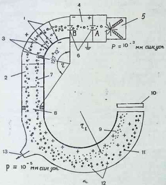
1.1-а расм. Демпстер масс-спектрографи.
