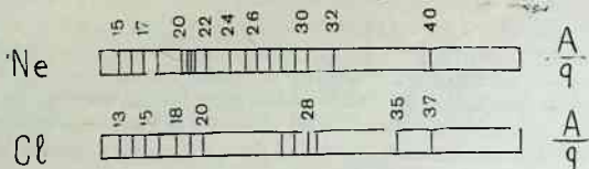
1.1-б расм. Неон ва хлор масс-спектрограммаси. 20—22 Ne изотопи; 35, 37 — Cl изотопларининг излари; 28— углерод нонларининг излари (спектрини даражалаш учун фойдаланилган); 17,5; 18,5 — Cl изотопларининг икки зарядли нонлари излари; 13—18, 24—32; 40 — аралашма нонлар излари.
