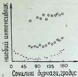
1.20-расм. Нейтронларнинг протонларда сочилиш бурчак тақсироти. Юқоридаги нуқта-лар 48 МэВ, ўртада 40 МэВ ва пастда 150 МэВ энергияли нейтронлар учун.
