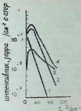
7.3-расм. Қосмик нурлар тўра компоненталарининг ҳавода ютилиши. 1— ядрвий актив компонента. 2— электрон-фотон компонента. 3— мюон компонента. 4— қосмик нурлар тўра интенсивлиги. Ҳаво қалинлигини кўрсатувчи узунлик бирлиги атмосферанинг юқори қатлаמידан бошлаб ўлчанган.
