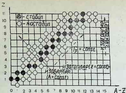
1.2-расм. Сегре диаграммаси.
