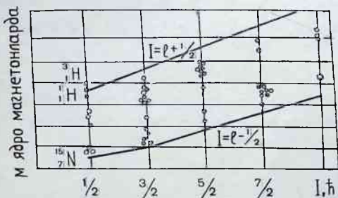
1.8-расм. Тоқ протонли ядроларнинг магнит momenti.
