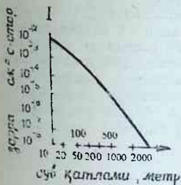
7.2-расм. Қосмик нурлар қаттиқ компонентасининг сувда ютилиши.
