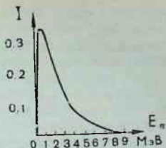
5.8-расм. Уран-235 нинг бўлинишида ҳосил бўлган нейтронлар энергетик спектри.
