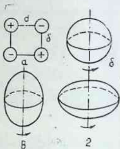
1.14-расм. а — электр квадруполь; б — сферик ядро; в — мусбат квадруполь моментли ядро; г — манфий квадруполь моментли ядро.
