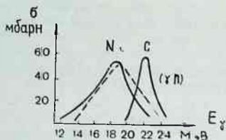
5.5-расм. Никель ва кўмир ядроларида қўзғатиладиган гигант резонанс қўзғалиш функциялари эғри чизиги.
