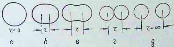
5.9-расм. Томчи моделига асосан ядронинг бўлиниши.
