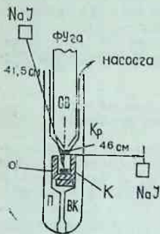
3.18-расм. Ву тажрибасининг схемаси.
