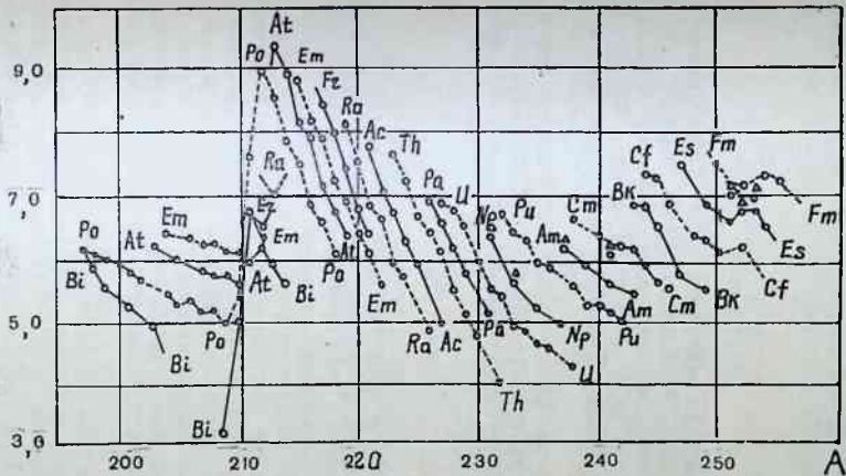
3.10-расм. Альфа-емирлиш энергиясининг альфа-радиоактив ядронинг масса сонн билан боғланши.
