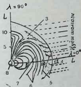
7.5-расм. а) Ернинг Қуёшга қараган томонида магнитосферанинг схемаси; б) магнитосферанинг меридиан бўйлаб кесими. 1,5— магнитопауза; 2,4— зарб тўлақини; 3— қолинич нуқта; 5— магнит майдон куч чизиқлари; 7— ташқи радиацион минтақа соҳаси; 8— Ер; 9— ўтувчи (турбулент) қатлам.
