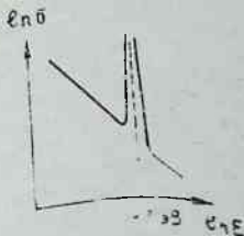
5.1-расм. Уран-238 да нейтронлар ютилиш кесимининг нейтрон энергиясига боғлиқ равишда резонанс ўзгариши.
