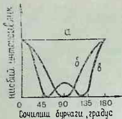
1.19-расм. Нуклонларнинг нуклонларда сочилиш бурчак тақсироти. а) соф S -тўлқин учун; б) соф D -тўлқин учун; в) соф P -тўлқин учун.
