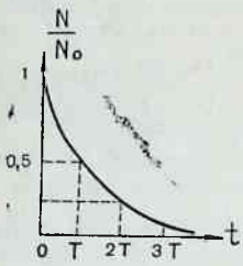
3.1-расм. Радиоактив радон ядролар сонининг вақт ўтиши билан ўзгариши.
