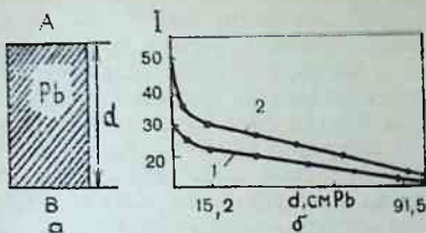
7.1-расм. а) телескоп схемаси; б) космик нурларнинг юмшоқ ва қаттиқ компонентасини кўрсатувчи эгри чизик. 1— денгиз сатҳида, 2— денгиз сатҳидан 3200 м баландликда.
