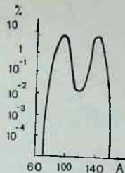
5.6-расм. Уранининг бўлинишида ҳосил бўлган ядроларнинг масса бўйича тақсимланиши.
