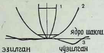
2.3-расм. Ташқи нуклонлар сонига қараб ядро потенциалининг ўзгариши.
