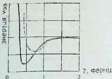
1.18-расм. Спинлари антипараллел бўлган икки протон орасидаги кучли ўзаро таъсирнинг потенциал энергияси.
