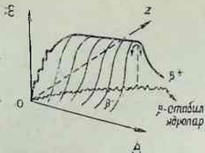
1.5-расм. Энергетик сирт.
