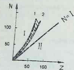
3.4-расм. Ядроларнинг нейтрон-протон диаграммаси.
