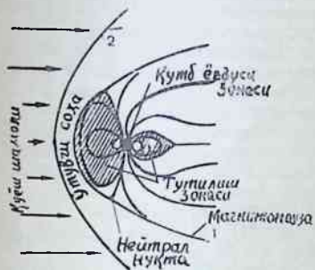
7.5-расм. а) Ернинг Қуёшга қараган томонида магнитосферанинг схемаси; б) магнитосферанинг меридиан бўйлаб кесими. 1,5— магнитопауза; 2,4— зарб тўлақини; 3— қолинич нуқта; 5— магнит майдон куч чизиқлари; 7— ташқи радиацион минтақа соҳаси; 8— Ер; 9— ўтувчи (турбулент) қатлам.
