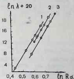
3.9-расм. Гейгер-Нетолл қонуни графиги
