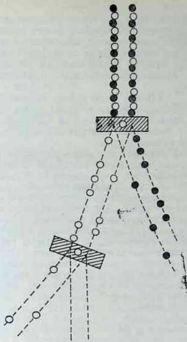
1.21-расм. Протонларнинг қутбланишига доир тажриба схемаси.
