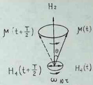
1.11-расм. Кучсиз ўзгарувчан H_1 майдон таъсирида магнит момент билан H_2 майдон йўналиши орасидаги \theta бурчакнинг ўзгариши.
