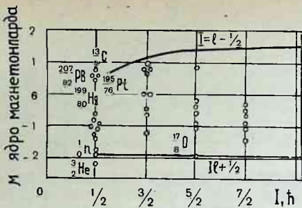
1.9-расм. Тоқ нейтронли ядроларнинг магнит моменти.
