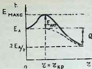
5.11-расм. Ядро энергиясининг r га қараб ўзгариши.
