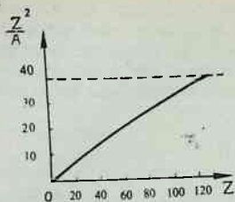
5.10-расм. Бўлиниш параметрининг Z га қараб ўзгариши.
