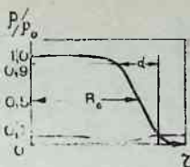
1.4-расм. Ядро заряд зичлиги тақсмотининг Ферми модели.
