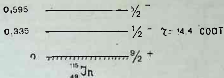
3.20-расм. 115 In ядросининг сатҳлар схемаси.
