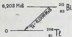
3.6-расм. Висмут-212 нинг емирилиш схемаси.
