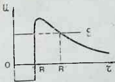
1.3-расм. Альфа-заррани ядро ичида тўтиб турувчи потенциал майдон.
