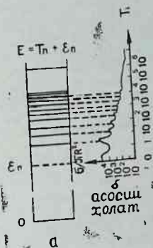
5.2-расм. Нейтрон ютилиш кесими билан ядро энергетик сатҳлари орасидаги боғланиш: а — энергетик сатҳлар схемаси; б — комплаунд ядро ҳосил бўлиш ҳиссининг энергияга боғлиқ равишда ўзгариши.
