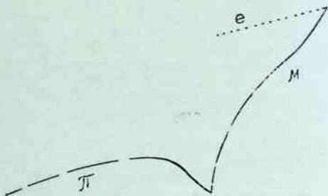
6.1-расм. \pi \rightarrow \mu \rightarrow e парчаланиш.
