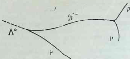
6.3-расм. \Lambda^0 -гипероннинг парчаланиши.
