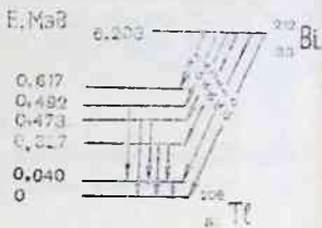
3.7-расм. Альфа-емирилиш нозик структураси.
