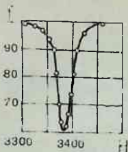
1.12-расм. Li учун резонанс эгри чизик.
