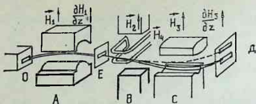
1.10-расм. Раби тажрибасининг схемаси.
