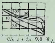
4.7-расм. 2,5; 10; 50 ва 500 МэВ энергияли электроларнинг радиацион нурланиш спектри.
