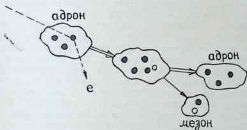
6.7-расм. Юқори энергияли электрон билан адрон бомбардимон этилганда мезоннинг ҳосил бўлиши.
