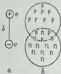
1.13-расм. а — электр диполь; б — протонлари нейтронларга нисбатан силжиган ядро.
