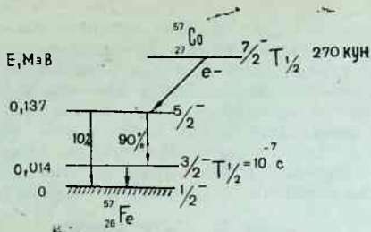
3.22-расм. ^{57}_{27}\text{Co} Сонинг парчаланиш схемаси.
