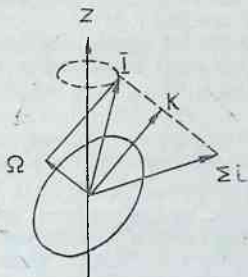
1.15-расм. Ядро хусусий квадруполь моментининг нейтрон (ёки протон) сонига қараб ўзгаршини.
