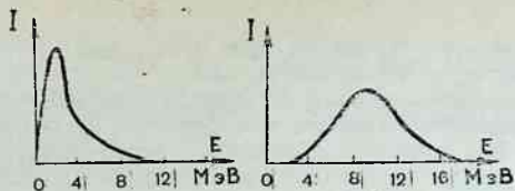
5.3-расм. Қўзғатилган ҳолатдаги ораліқ ядродан чиқувчи нуклонларнинг энергетик спектри: a — нейтронлар учун; b — протонлар учун.
