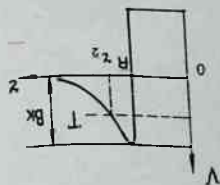
5.4-расм. Зарядланган зарра билан ядронинг Кулон таъсир потенциал
