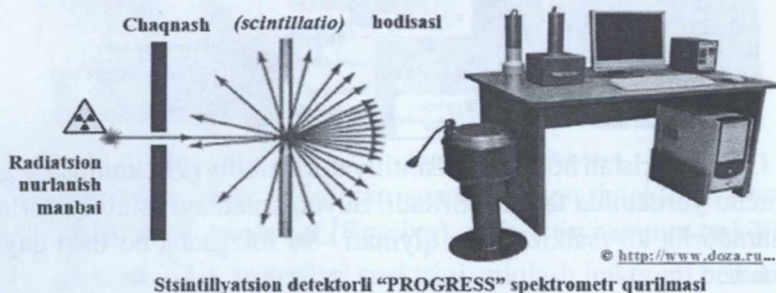
Stintillyatsion detektorli "PROGRESS" spektrometr qurilmasi
