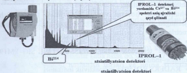
«InSpector-1000» spektrometri (AQSH)
