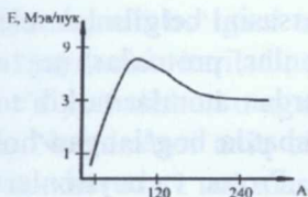
1-rasm. Solishtirma bog‘lanish energiyasi( \epsilon )ning atom massasi(A)ga bog‘liqlik grafiqi.
