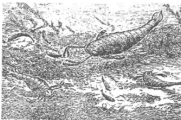
II-рaсм. Silur dengizi tubida tarqalgan 3 metrli qisqichbaqa — dengiz yirtqichlari.
