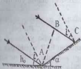
3.6 - rasml. Og'ma sirtga tushuvchi to'g'ri quyosh radiatsiyasini aniqlash
