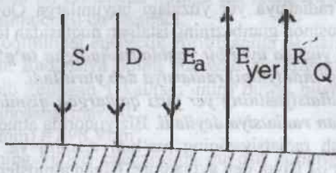
3.1-rasm. Atmosferadagi nurlanish oqimlari yo'nalishlari
