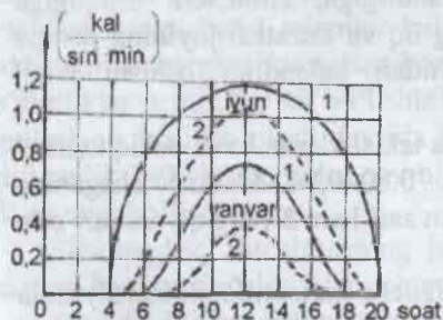
3.5-rasm. Toshkent shahrida quyosh nurlariga tik (1) va gorizontal joylashtirilgan yuza (2) ga tushyotgan to'g'ri radiatsiya energetik yoritilganligining sutkalik o'zgarishi
