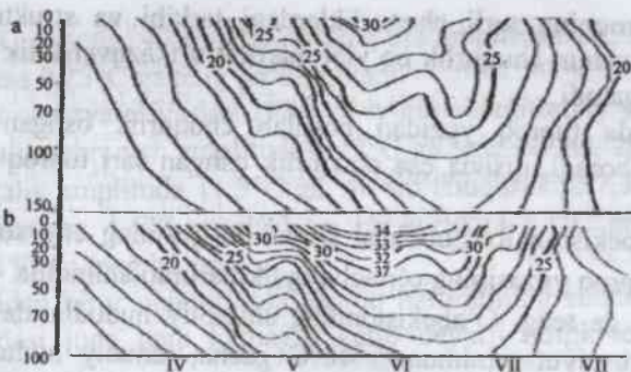
4.2 - rasm. Bo'z tuproqli yerning termoizopletlari a – nazoratdagi tuproq, b – mulchalangan uchastka.
