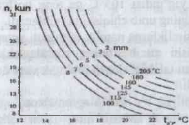
14.2-rasm. G'o'za chigitini ekish-unib chiqish davri davomiyligi ( n ) ning, o'rtacha sutkalik havo haroratiga ( t_{0,r} , °C), samarali havo haroratlar yig'indisi ( \Sigma t_s ) va tuproqning 0–5 sm chuqurlikdagi namligiga bog'liqlik nomogrammasi
