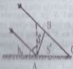
3.4-rasm. To'g'ri quyosh radiatsiyasining quyosh nurlariga tik qo'yilgan yuzadagi ( S ) va gorizontal yuzadagi ( S^l ) energetik yoritilganliklari
