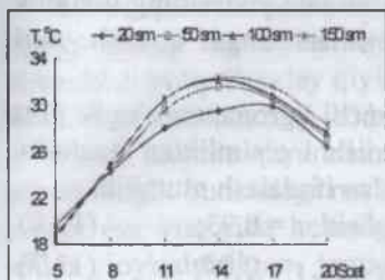
12.4-rasm. Sholi dalasida iyun oyida har xil balandlikda kunduzgi havo haroratining o'zgarishi
