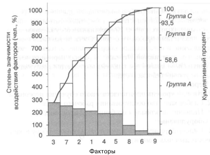
Рис. 1.3. Простая и кумулятивная диаграммы Парето
