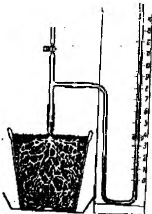
50-чизма. Симоб монометри билан илдиз босимини ўлчаш.
