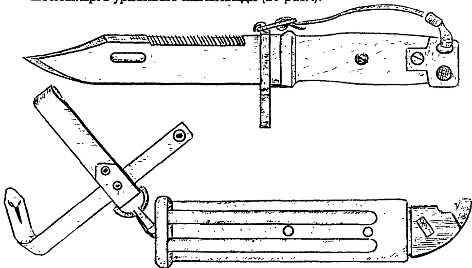
21-расм. АКМ автоматининг милтиқ найза-пичоғи ва унинг қини
