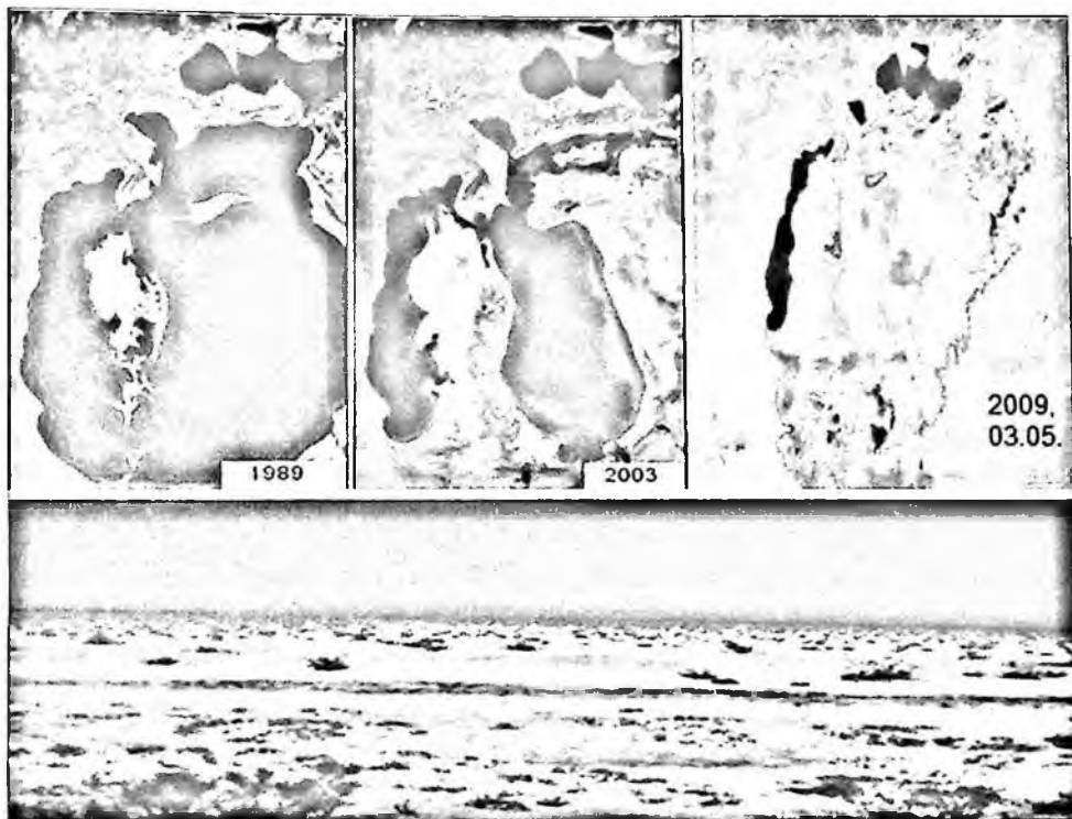
2.1-расм. Орол денгизи ва қуриб қолган денгиз тубининг ер йўлдошидан олинган суратлари.
