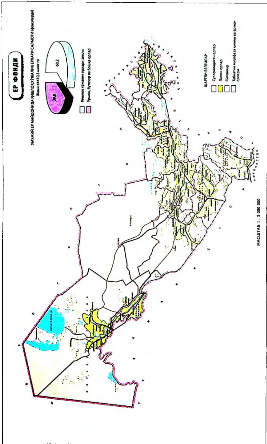
3.1-расм Ўзбекистон Республикасида ер фонди харитаси. Манба: Ўзбекистоннинг экологик атласи, МВССО РУз., ЎзР Дағи ЮНЕСКО ваколатхонаси. Тошкент, 2007.
