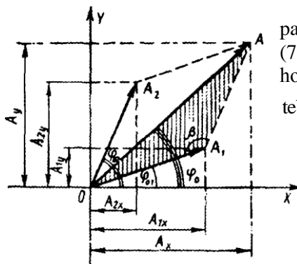
7.7- rasm. doira-viy chastotaga ega bo'lgan garmonik harakat bo'lib, quyidagicha ifodalanadi:
