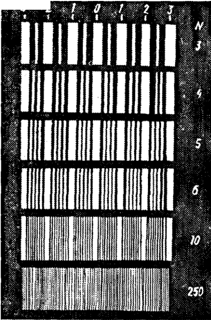
24.15- rasm. intervalda joylashgan bosh maksi-mumlardan foydalanishga intiladi. Difraksion panjaraga oq
