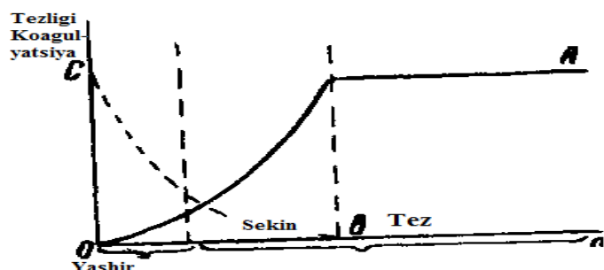
11.7 - rasm Koagulyatsiya tezligi (OA) va \zeta - potensial (SV) ning elektrolit konsentratsiyasiga bogʻliqligi.
